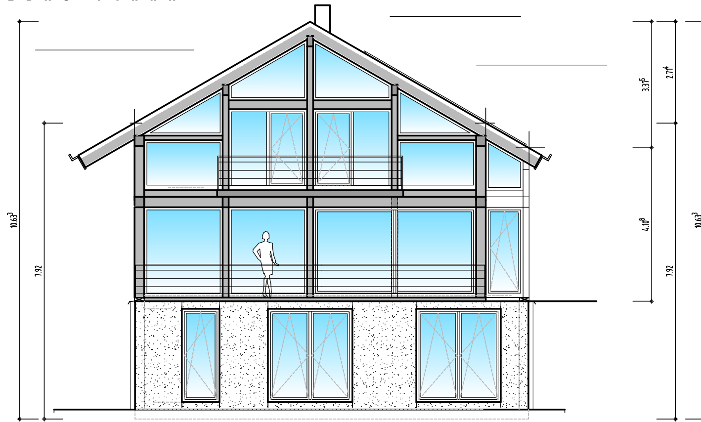
ANSICHT WEST
