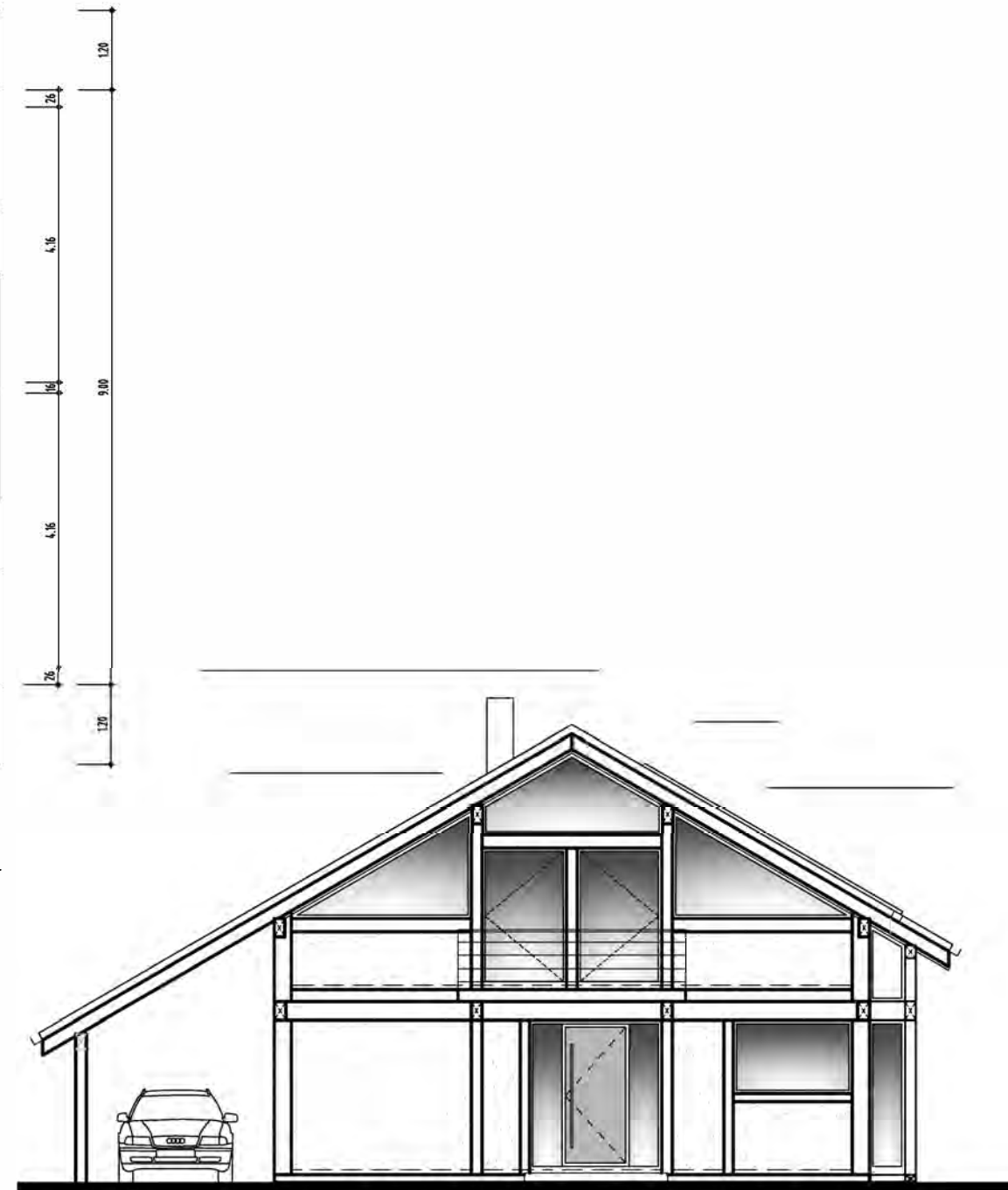
ANSICHT VON WESTEN MIT CARPORT
