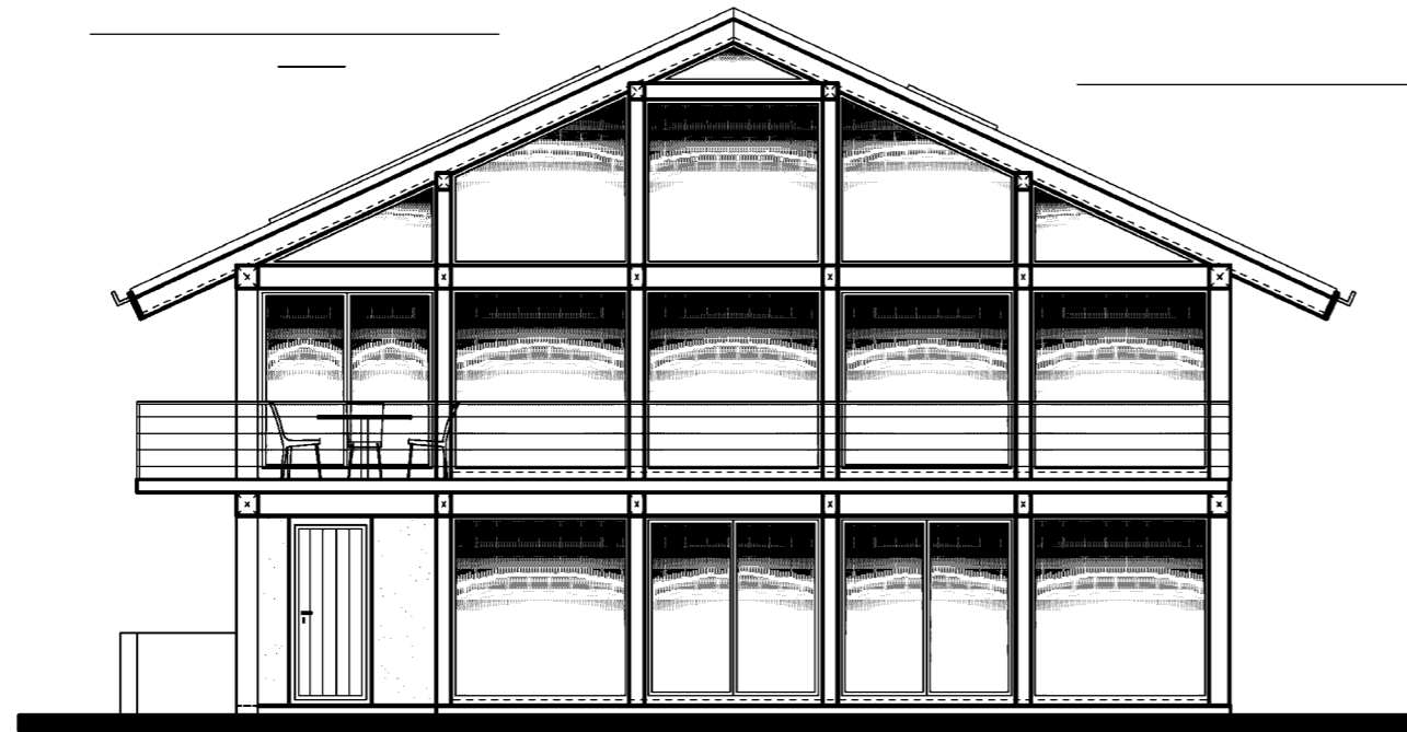
ANSICHT TALSEITE
