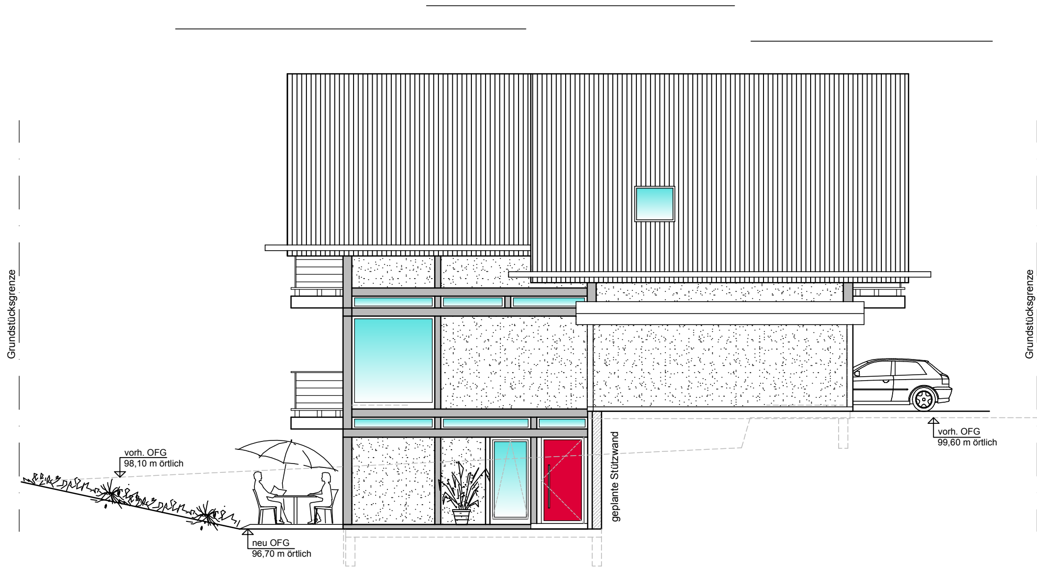
ANSICHT NORD WEST
